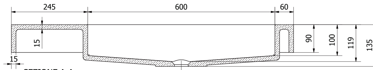
SEZIONE A-A
