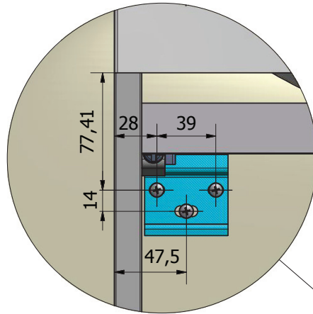
DETTAGLIO A
