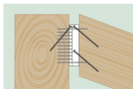
Anschluss geneigt (Seitenansicht)
