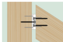
Anschluss schräg (Draufsicht)
