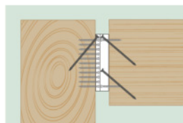
Anschluss 90° (Seitenansicht)
