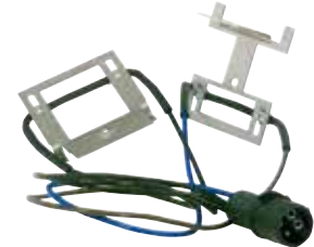
Abgassensor • Passend für Vaillant: VC/VCW • Ref.-Nr.: 25-3537
