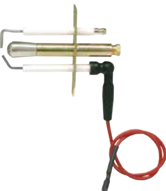
Viessmann • Passend für Viessmann Vitogas 100, Typ GS1/A/B, 11 bis 144 kW, Vitogas 050, Typ GSOA/B, 29 bis 60 kW, Vitogas 300, Typ GS3, Atola-RN, Typ ARN, AVB, Litola, Typ LV, VB, LVR Rexola-triferral, Typ RTF • Ref.-Nr.: 7822652
