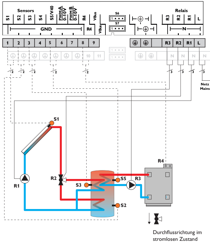
Hydraulikvariante 1
