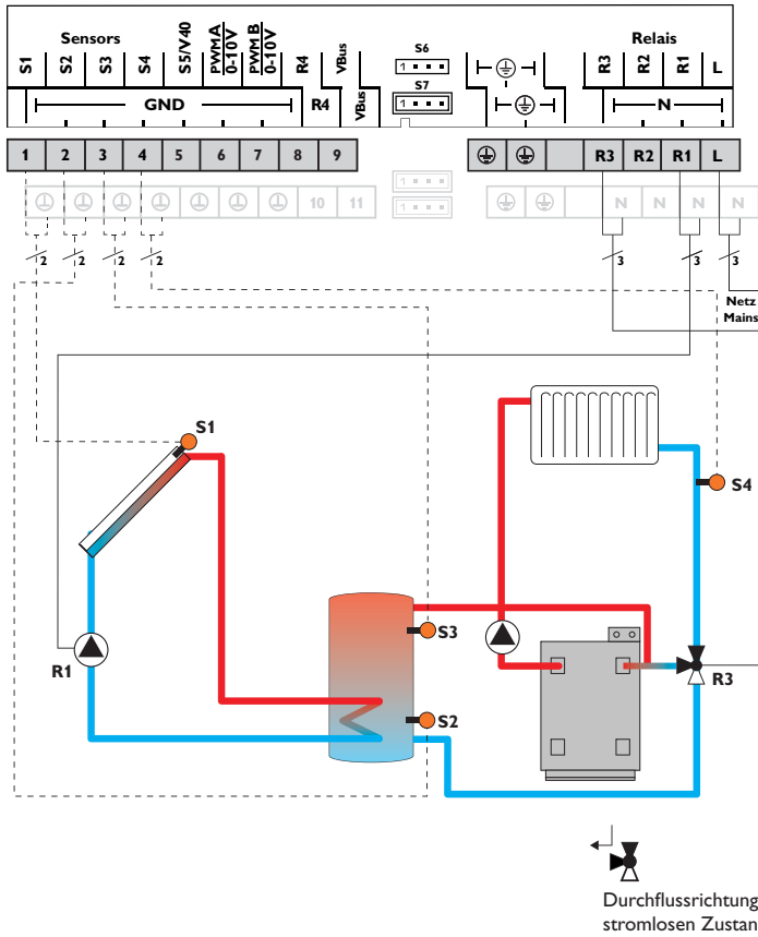
Hydraulikvariante 1
