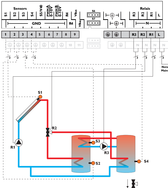
Durchflussrichtung im stromlosen Zustand
