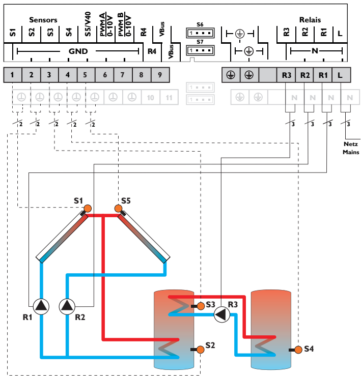
Hydraulikvariante 1
