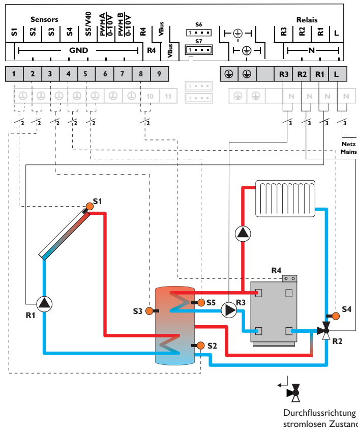
Hydraulikvariante 1
