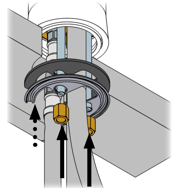
Montaggio Lavello - Assembly sink mixer
