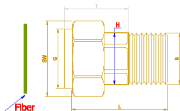
ΣÉT Υδρομέτρου Water Meter Connector
